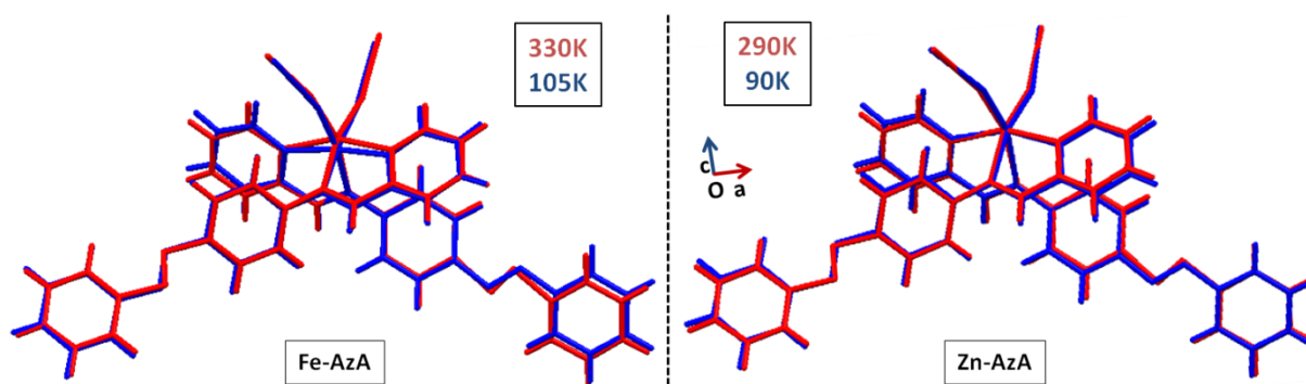
Figure 25 Superpositions des structures moléculaires selon l'axe b_2 à gauche, du Fe-AzA à 330K (en rouge) et à 105K (en bleu), et à droite du Zn-AzA à 290K (en rouge) et à 90K (en bleu).
