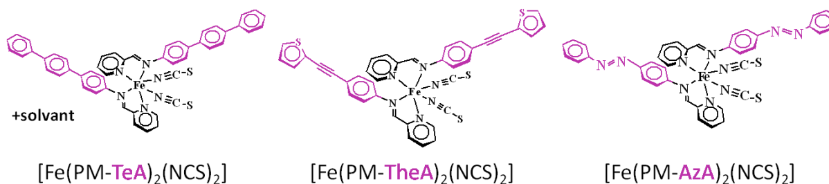
Figure 16 Schémas moléculaires des trois complexes [\text{Fe}(\text{PM-TeA})_2(\text{NCS})_2].\text{MeOH} , [\text{Fe}(\text{PM-TheA})_2(\text{NCS})_2] et [\text{Fe}(\text{PM-AzA})_2(\text{NCS})_2] étudiés dans ce chapitre pour tester l'outil « mosaïcité » du logiciel Denzo. Les ligands TeA, TheA et AzA qui distinguent ces complexes sont colorés en rose.
