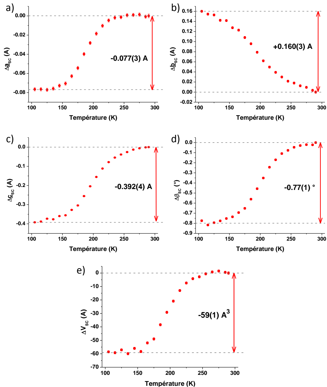
Figure 12 Variations réelles du volume ( \text{Å}^3 ) et des paramètres de maille ( \text{Å} ) du Fe-AzA corrigées de la contribution thermique. a) \Delta a_{\text{sc}}(\text{T}) , b) \Delta b_{\text{sc}}(\text{T}) , c) \Delta c_{\text{sc}}(\text{T}) , d) \Delta \beta_{\text{sc}}(\text{T}) , e) \Delta V_{\text{sc}}(\text{T}) . Seuls les effets de la conversion de spin sont donc représentés.
