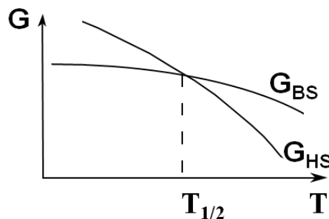
Figure 5 Allure des évolutions des énergies de Gibbs des systèmes HS et BS en fonction de la température dans le modèle de gaz parfait de molécules à conversion de spin .
