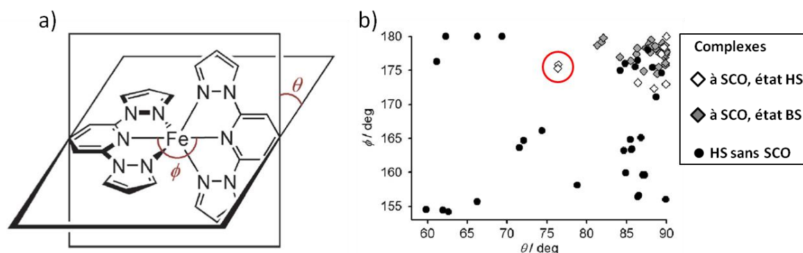
Figure 21 a) Représentation du cation [\text{Fe}(1\text{-bpp})_2]^{2+} et des deux angles \phi et \theta décrivant sa géométrie.
