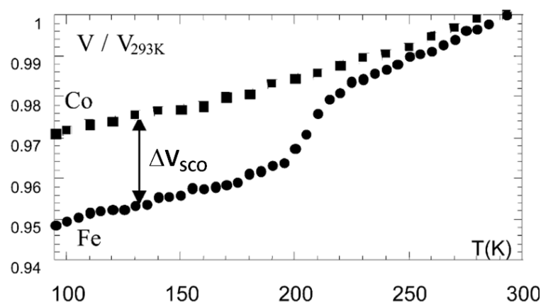
Figure 27 Evolution en fonction de la température du volume relatif des mailles des complexes isostructuraux [\text{Fe}(\text{PM-BiA})_2(\text{NCS})_2]\text{-II} (cercles) et [\text{Co}(\text{PM-BiA})_2(\text{NCS})_2] (carrés), et mise en évidence de \Delta V_{SCO, T} , variation volumique due à la SCO thermique [Guionneau 2002, 2004].
