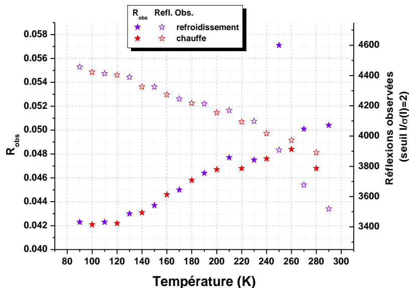
Figure 9 Graphe donnant l'évolution des affinements des 21 structures issues des 21 collectes du Zn-AzA (détails en annexe A-6). Les symboles pleins correspondent aux R_{obs} (échelle de gauche), les symboles creux aux nombres de réflexions observées (seuil : I/\sigma(I) \geq 2 ) (échelle de droite)
