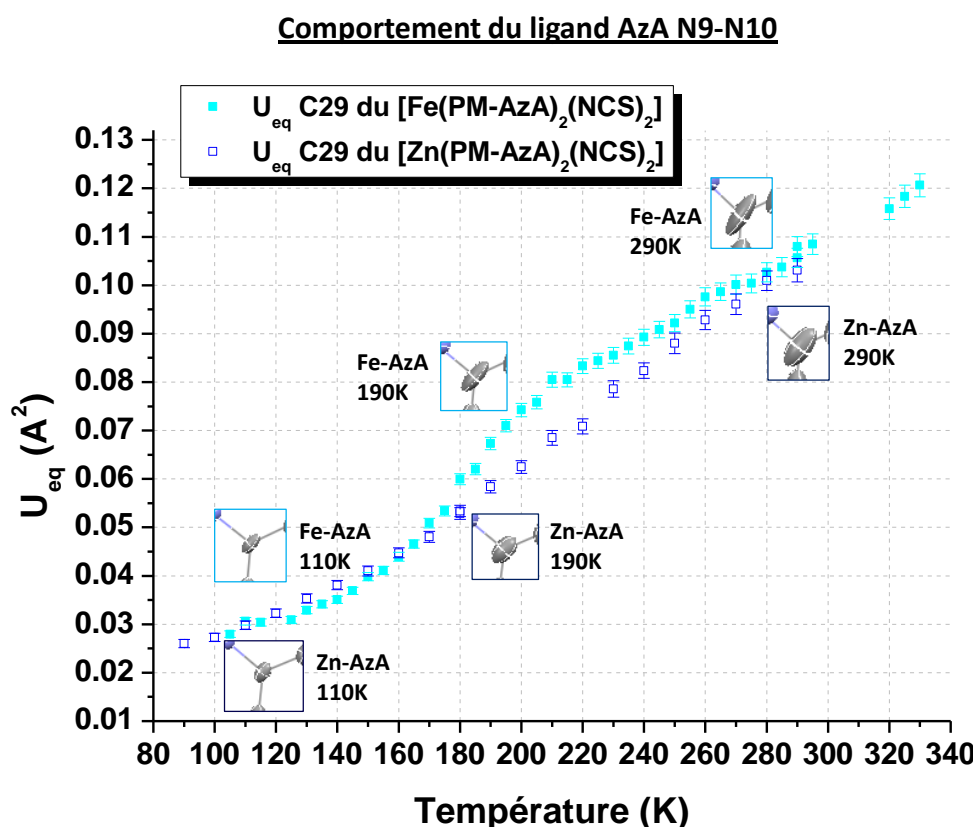
Figure 34 Comparaison des évolutions des paramètres de déplacement atomique isotropes U_{eq} des atomes de carbone C29 des molécules de Fe-AzA et Zn-AzA en fonction de la température, et représentation sous forme d'ellipsoïdes à 50% de probabilité de l'atomes C29 des deux complexes à différentes températures.
