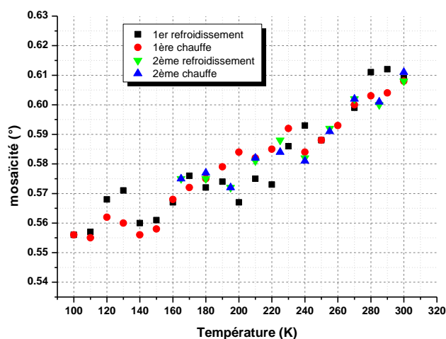
Figure A7-5 : Fe-TheA-II : Evolution de \mathcal{M} au cours de deux cycles thermiques.
