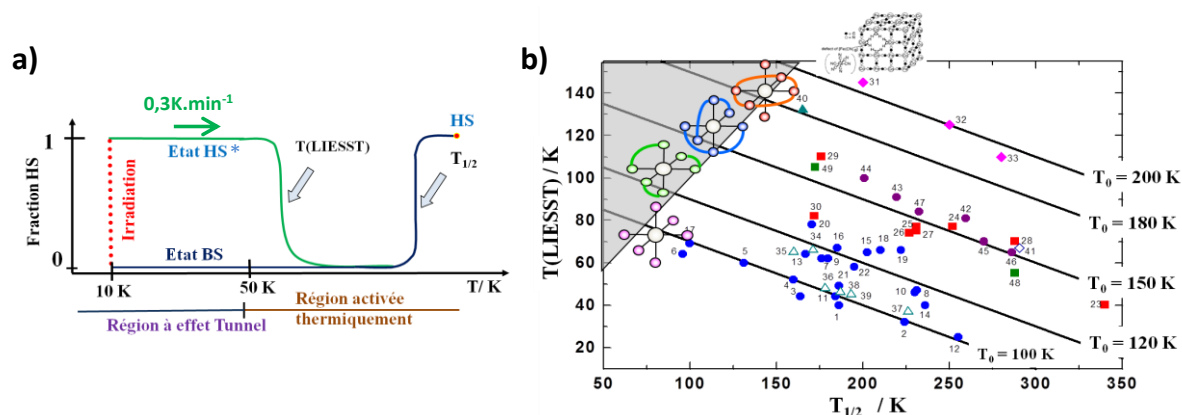
Figure 9 a) Principe de mesure de la T(\text{LIESST}) , b) Base de données T(\text{LIESST})/T_{1/2} et influence de la sphère de coordination sur la stabilité de l'état HS. Les données pour les lignes T_0 = 100\text{K} et 120\text{K} correspondent à des complexes aux ligands de faible denticité et sont rapportées dans la ref [Létard 1999]. La ligne T_0 = 150\text{K} résulte de la régression linéaire obtenue avec la famille [\text{Fe}(\text{bpp})_2]\text{X}_2 \cdot n\text{H}_2\text{O} , aux ligands tridentés [Marcén 2002]. La ligne T_0 = 200\text{K} est basée sur le travail de Hashimoto, portant sur des complexes s'organisant en réseaux tridimensionnels [Shimamoto 2002]. La zone grisée est sans sens car la T(\text{LIESST}) est inférieure, ou à l'extrême limite, égale à T_{1/2} (d'après [Létard 2006]).
