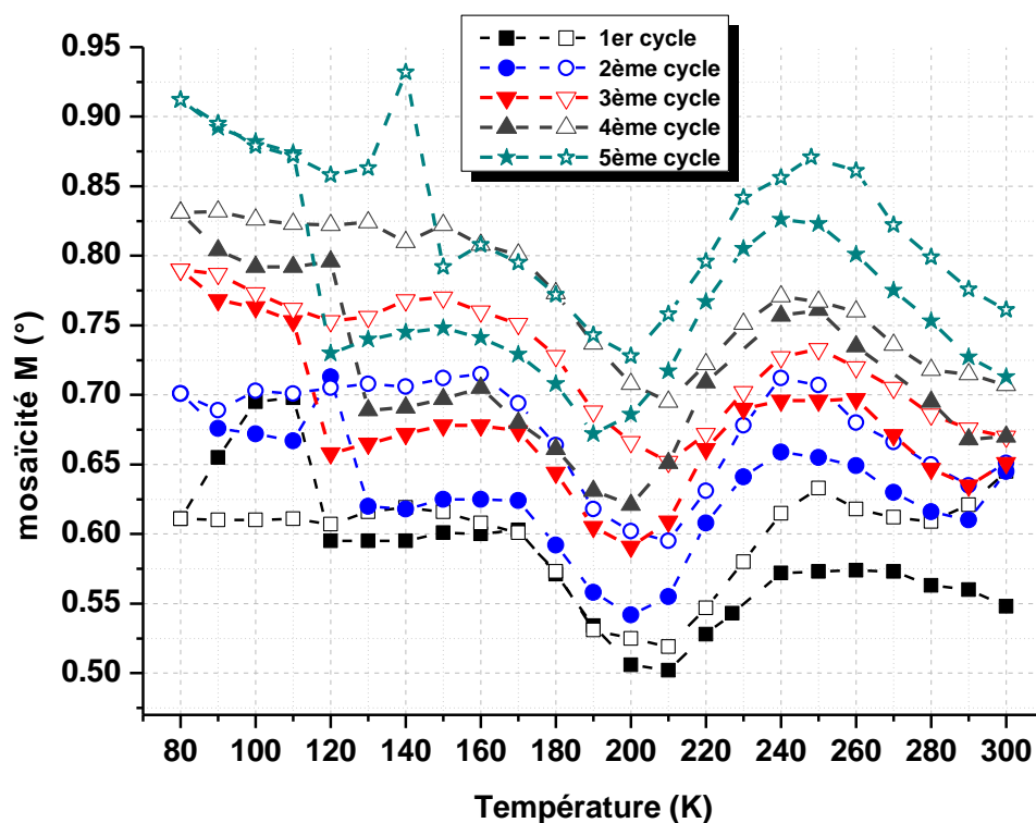
Figure 34 Fe-AzA : Evolution de la «mosaïcité» \mathcal{M} du cristal au cours des 5 cycles thermiques. Les symboles pleins représentent les refroidissements, les symboles vides, les chauffages. Les lignes en tirets lient les points expérimentaux sont des guides pour l'œil.
