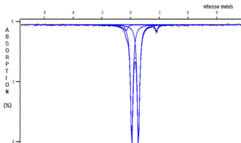
Figure A4-2 : Spectre Mössbauer d'une poudre de Fe-AzA à 4,2K
