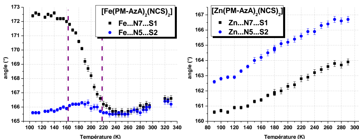
Figure 36 Suivi de l'évolution des angles MN5S2 et MN7S1 pour chacun des composés Fe-AzA (gauche), et Zn-AzA (droite).
