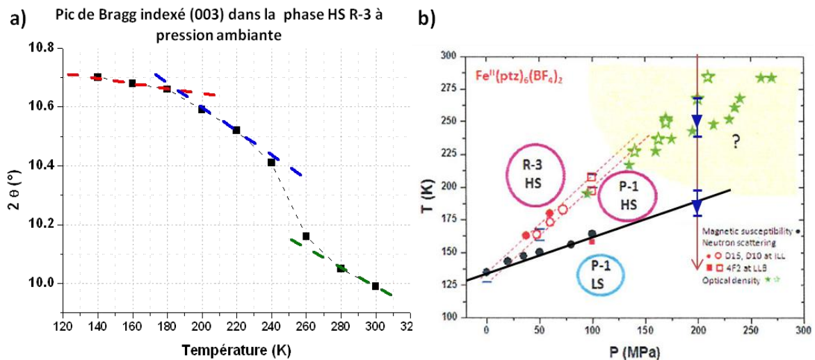
Figure 37 [\text{Fe}(\text{ptz})_6] (\text{}^{11}\text{BF}_4)_2 : a) Position en 2\theta du maximum du premier pic du diffractogramme (indexé (003) dans la phase HS R-3 sous pression ambiante) sous 200 MPa en fonction de la température. La courbe en pointillés noirs liant les points expérimentaux est un guide pour l'œil. Les trois régimes de déplacement du pic sont mis en évidence par des segments en pointillés colorés.
