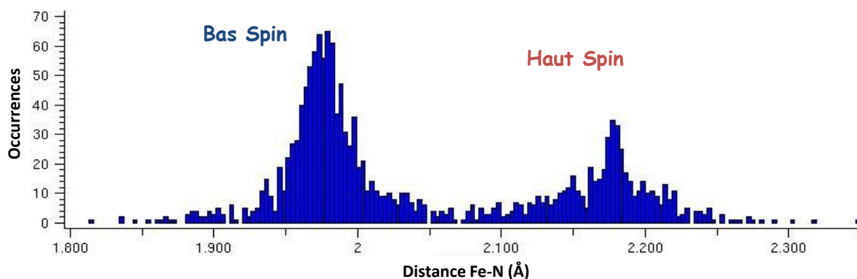
Figure 16 Histogramme des distances Fe-N des complexes de fer dont la sphère de coordination est composée de six atomes d'azote. Seules les 1243 structures de la Cambridge Structural Database résolues sur monocristal sont considérées (recherche CSD effectuée en novembre 2012).
