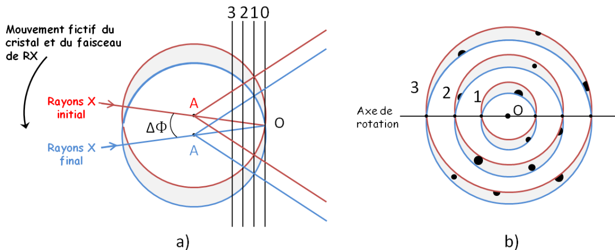
Figure 5 Schémas illustrant la méthode de rotation.
