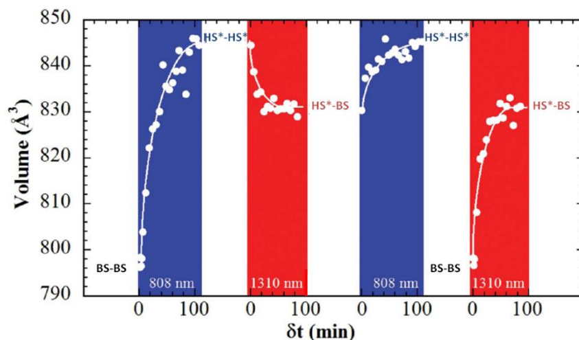
Figure 10 Evolution à basse température du volume de la maille cristalline directement lié à l'état de spin du complexe dinucléaire [\text{Fe}(\text{bt})(\text{NCS})_2]_2(\text{bpym}) , en fonction du temps et sous différentes excitations lumineuses. L'irradiation à 808nm (bleu) photo-induit la phase HS*-HS* quel que soit l'état initial du complexe, celle à 1310nm photo-induit la phase HS*-BS [Trzop 2007].
