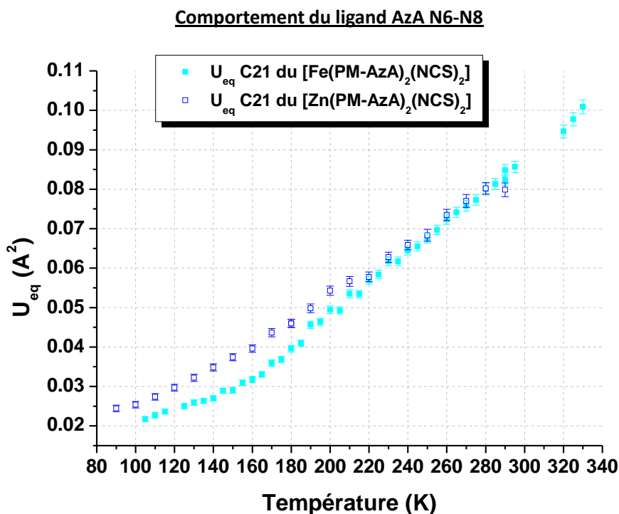
Figure 32 Comparaison des évolutions des paramètres de déplacement atomique isotropes U_{\text{eq}} des atomes de carbone C21 des molécules de Fe-AzA et Zn-AzA en fonction de la température.
