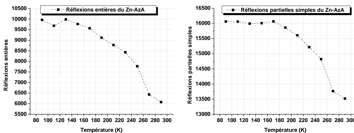
Figure 36 Zn-AzA : Evolution des nombres de réflexions entières (à gauche) et partielles simples (à droite) considérées par le logiciel de calcul de la « mosaïcité » \mathcal{M} au cours d'un refroidissement.
