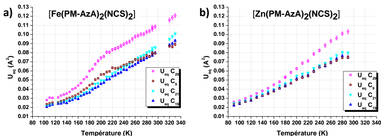
Figure 31 Evolution des paramètres de déplacement atomique isotropes U_{\text{eq}} ( \text{\AA}^2 ) des atomes de carbone C19 C21 C9 et C29 des deux groupements AzA des molécules de Fe-AzA (a) à gauche) et Zn-AzA (b) à droite) en fonction de la température.
