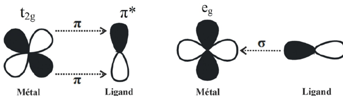
Figure 15 Illustration d'une interaction \pi (à gauche) et d'une interaction \sigma (à droite).
