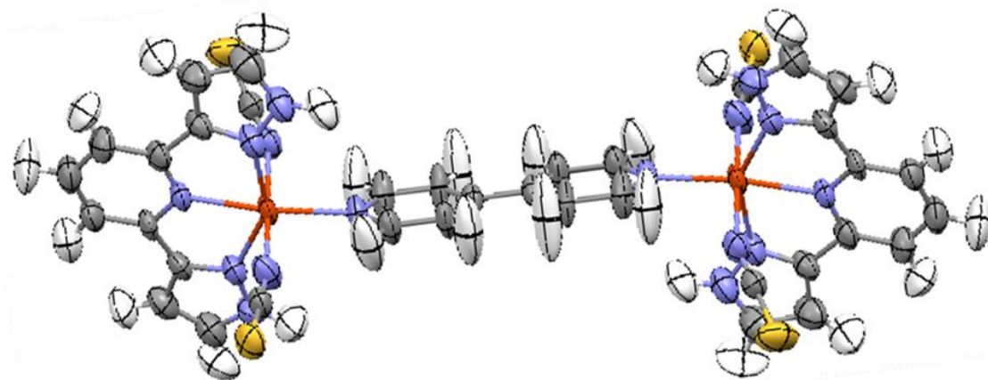
Figure 33 dinNCS : Structure moléculaire résolue par diffraction des neutrons sur VIVALDI à température ambiante avec des facteurs de déplacement atomique anisotrope à 50% de probabilité. Cette structure met en évidence des ellipsoïdes de déplacement anisotrope particulièrement allongés pour les atomes d'hydrogènes des cycles aromatiques, et dans une moindre mesure pour les atomes de carbone de ces cycles.
