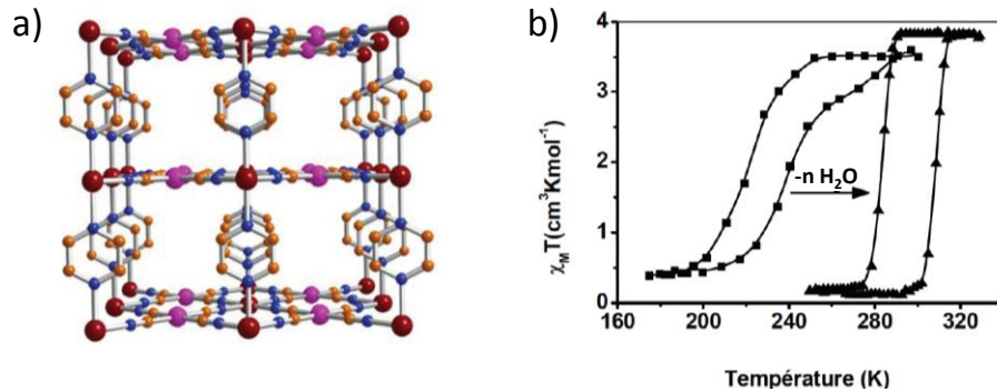
Figure 25 a) Représentation de la structure du complexe [Fe(pyrazine){Pt(CN) 4 }]·nH 2 O b) Evolution du produit \chi_M T en fonction de T en refroidissement et chauffe du complexe hydraté et déshydraté (adaptée de [Bonhommeau 2005]).
