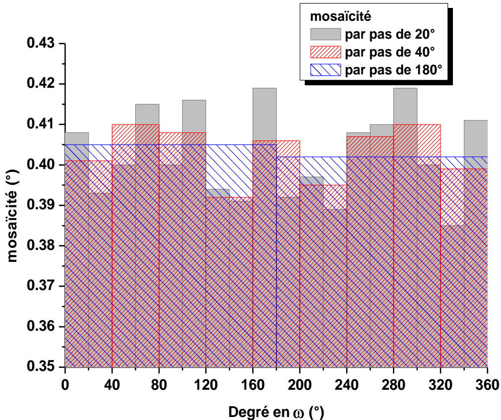
Figure 9 Mosaïcité \mathcal{M} pour un scan complet de 360° en \omega , traité par pas de 20° (gris), de 40° (hachuré en rouge), et de 180° (hachuré en bleu).
