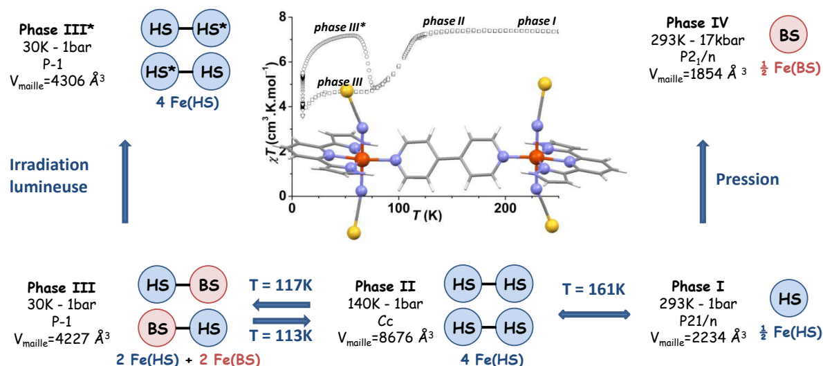
Figure 25 dinNCS : Schéma résumant le diagramme de phase, avec dénomination des phases connues en température, pression et irradiation lumineuse, températures de transition, groupes d'espace et états de spin correspondants [Fedaoui 2008, Kaiba 2010, Shepherd 2012].
