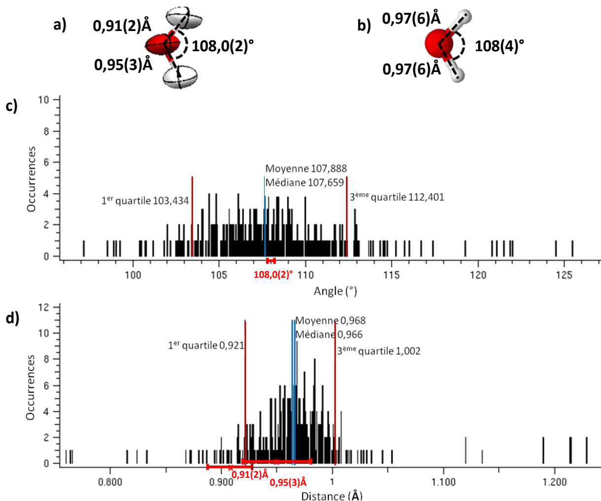
Figure 16 a) Représentation de la molécule d'eau résolue par diffraction des neutrons dans le complexe [\text{Fe}(\text{L}_{222})(\text{CN})_2] \cdot \text{H}_2\text{O} à 240K , b) représentation de la molécule d'eau moyenne des structures de la CSD résolues par diffraction de neutrons, c) histogramme des angles HOH des molécules d'eau des structures de la CSD résolues par diffraction des neutrons d) histogramme des distances O-H des molécules d'eau des structures de la CSD résolues par diffraction des neutrons (critères de recherche : structures résolues par diffraction des neutrons sur monocristal (146 résultats) et poudre (4 résultats)). Pour les histogrammes c) et d) sont donnés le premier quartile, le second ou médiane, le troisième, la moyenne des valeurs, et enfin les valeurs correspondant à la molécules d'eau du [\text{Fe}(\text{L}_{222})(\text{CN})_2] \cdot \text{H}_2\text{O} sont situées sur ces distributions.
