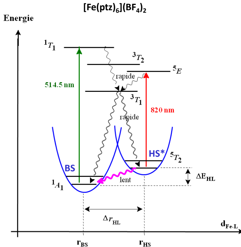
Figure 7 Diagramme énergétique du complexe [\text{Fe}(\text{ptz})_6](\text{BF}_4)_2 , avec illustration du phénomène LIESST par irradiation à 514,5 nm depuis l'état BS (flèche verte) et relaxations, et reverse-LIESST par irradiation à 820 nm depuis l'état HS* (flèche rouge) et relaxations. La flèche rose représente la possibilité de relaxation \text{HS}^* \rightarrow \text{BS} par effet tunnel. D'après [Hauser 1986 et 1991].
