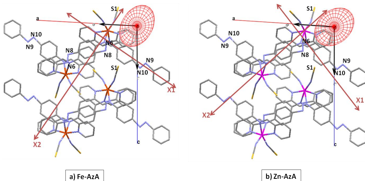
Figure 15 Superposition de la surface de dilatation obtenue à partir des coefficients de dilatation thermique [Cliffe 2012] et de l'arrangement cristallin selon l'axe b entre 260K et 290K pour le Fe-AzA (a) et pour le Zn-AzA (b).
