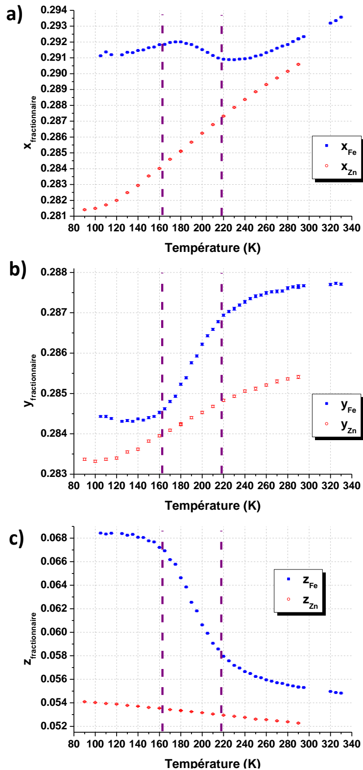
Figure 17 Mouvement de l'ion métallique \text{Fe}^{\text{II}} ou \text{Zn}^{\text{II}} au cours du ou des cycles thermiques, en coordonnées fractionnaires.
