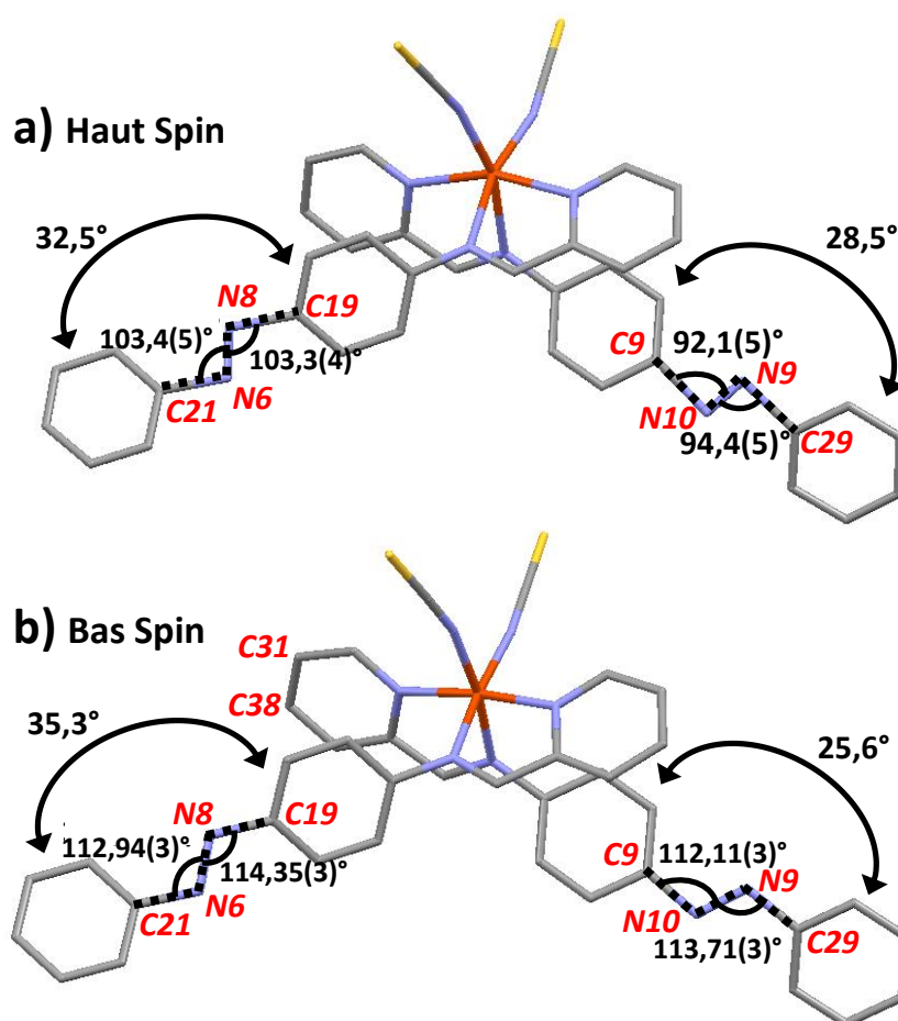
Figure 6 Représentation de la molécule de Fe-AzA dans les états HS à 293K (a) et BS à 110K (b). Les mesures des angles CNN des groupements AzA sont données [Guionneau 1999], ainsi que la torsion des bras AzA.
