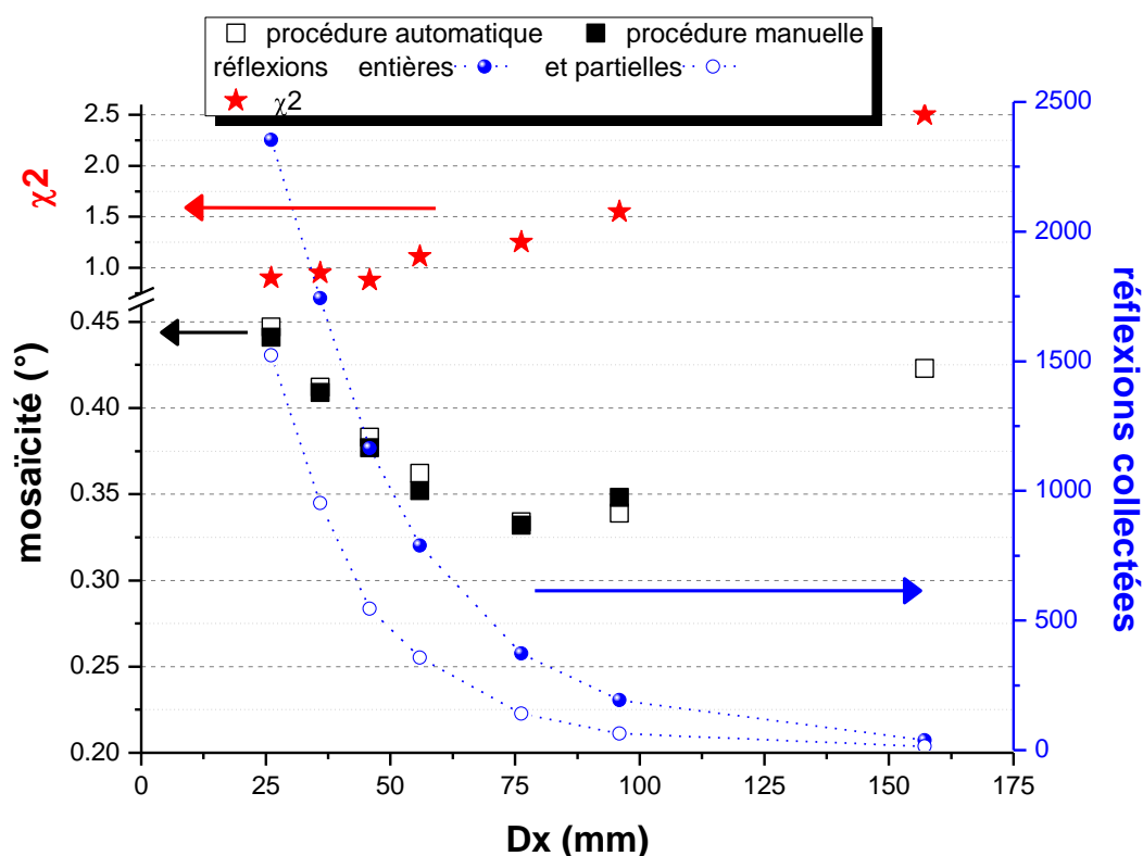
Figure 8 Valeurs de «mosaïcité» obtenues avec les deux procédures, automatique et manuelle, pour différentes valeurs de Dx. Les barres d'erreurs sur \mathcal{M} sont de l'ordre de la taille des symboles. Pour chaque mesure sont donnés les nombres de réflexions acquises entièrement sur une unique image (réflexion entières) et acquises sur deux images (réflexions partielles simples), ainsi que la valeur de \chi^2 . La procédure manuelle ne renvoie pas d'estimation de \mathcal{M} pour Dx >150mm, par manque de données.
