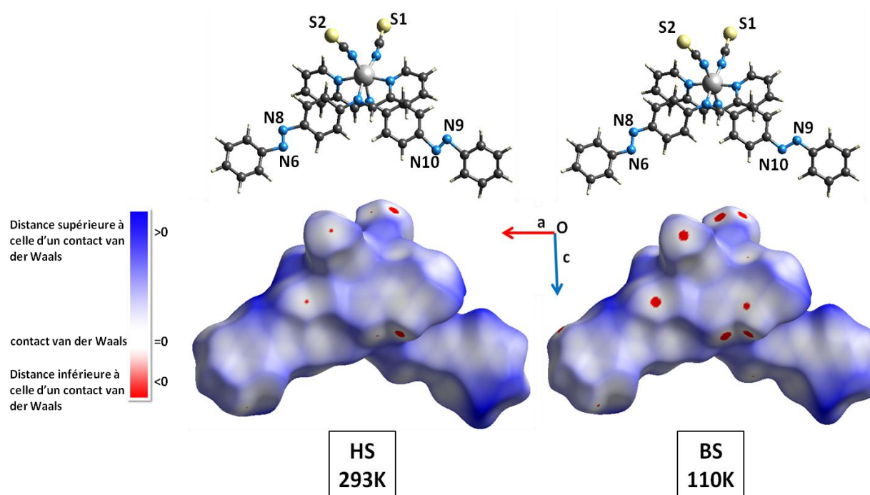
Figure 5 Vue selon \underline{b} des structures moléculaires (en haut) et des surfaces d'Hirshfeld (en bas) des molécules HS à 293K (à gauche) et BS à 110K (à droite) de Fe-AzA obtenues avec le programme CrystalExplorer. Les zones rouges correspondent aux distances intermoléculaires inférieures à la somme des rayons de van der Waals, les zones bleues aux distances supérieures à la somme des rayons de van der Waals (les structures moléculaires utilisées sont publiées dans la Cambridge Structural Database [Guionneau 1999]).
