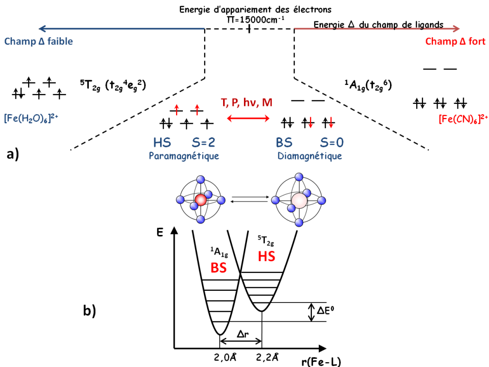
Figure 3 a) Représentation schématique du remplissage électronique des orbitales 3d d'un ion \text{Fe}^{\text{II}} en fonction de la force de son champ de ligand. b) Représentation schématique de l'évolution de la sphère de coordination du métal lors de la SCO et diagramme des niveaux d'énergie de l'ion dans les deux configurations de spin, HS et BS.
