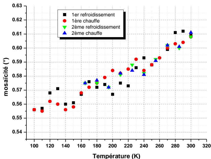
Figure 25 Fe-TheA-II : Evolution de la «mosaïcité» au cours des cycles thermiques.
