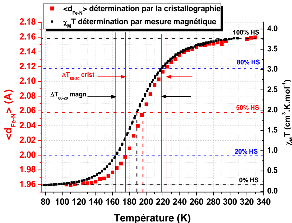
Figure 24 Superposition des évolutions en fonction de la température du produit \chi_M T de Fe-AzA déterminé par mesure magnétique sur monocristal (noir) (voir I-3-2-2) et du paramètre cristallographique \langle d_{\text{Fe-N}} \rangle (rouge) déterminé à l'aide de l'étude multi-structurale de Fe-AzA. L'évolution de \langle d_{\text{Fe-N}} \rangle est obtenue après déduction de l'effet thermique déterminé à l'aide de l'étude du Zn-AzA. Les domaines \Delta T_{80-20} dans lesquels la fraction HS varie entre 20% et 80% sont indiqués pour les deux déterminations.
