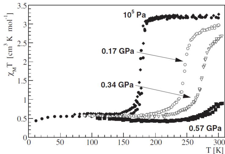
Figure 13 Evolution des variations de moment magnétique en fonction de la température du complexe [\text{Fe}(\text{phen})_2(\text{NCS})_2] sous différentes pressions [Gütlich 2004-b].
