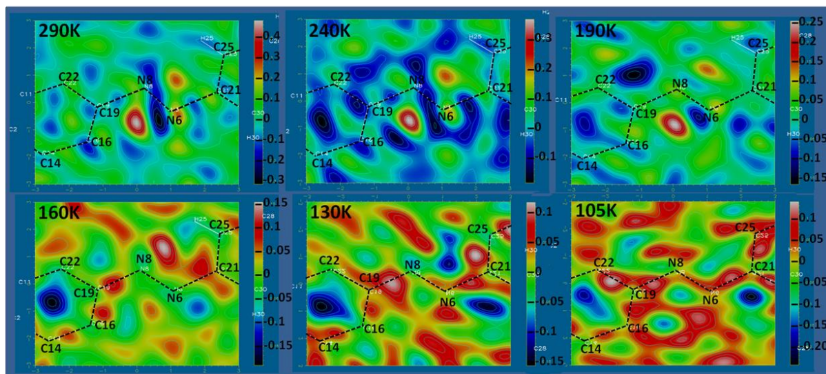
Figure 33 Cartes de densité de Fourier différence F_o-F_c dans le plan défini par les atomes C19, N6 et N8 du complexe Fe-AzA à différentes températures. Les zones rouges indiquent les résidus électroniques les plus importants. L'échelle de couleur à droite de chaque image donne l'intensité des résidus en électron.
