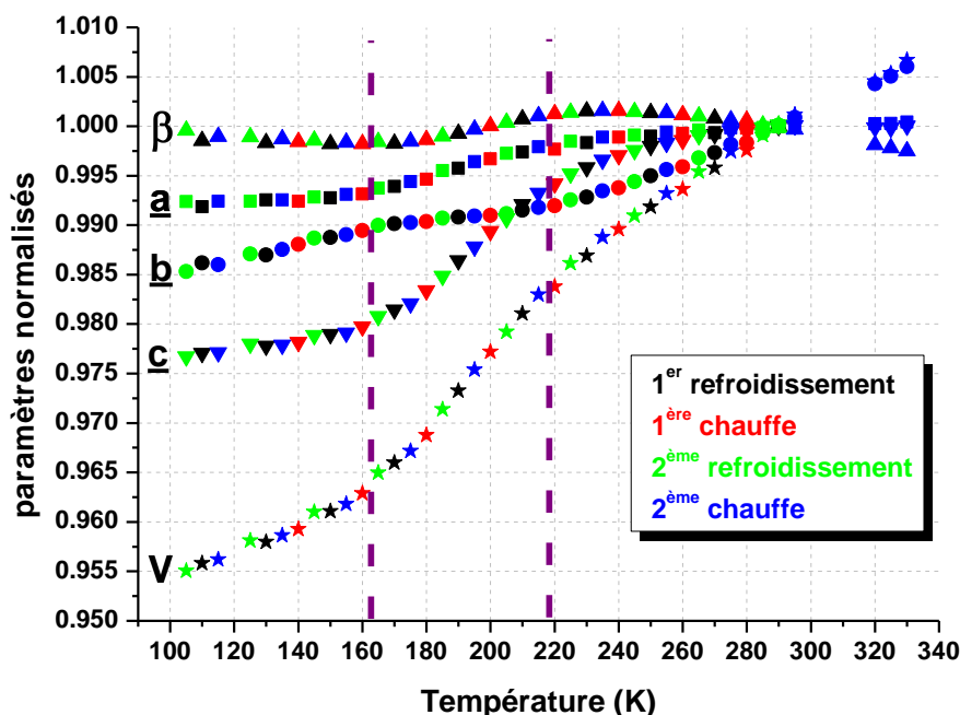
Figure 10 Evolution du volume (en \text{\AA}^3 ) et des paramètres de maille (en \text{\AA} ) du Fe-AzA au cours des deux cycles thermiques ( a : carrés, b : cercles, c : triangles pointe en bas, \beta : triangles pointe en haut, V : étoiles). Les paramètres sont normalisés par leur valeur à 290K. En noir : données issues de l'affinement des collectes du premier refroidissement, en rouge : celles issues de la première chauffe, en vert : deuxième refroidissement, en bleu : deuxième chauffe. Les deux droites verticales en tirets délimitent le domaine de température \Delta T_{80-20} déterminé par mesure magnétique sur monocristal.
