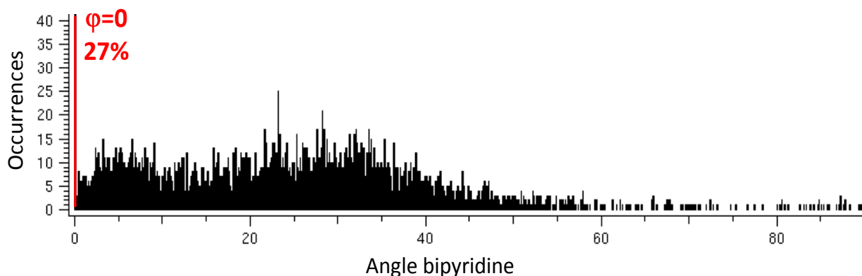
Figure 32 Histogramme des valeurs des angles entre les deux cycles des groupements bipyridines à partir des données de la Cambridge Structurale Data Base (critères de recherche : structures résolues sur monocristal ou poudre, par diffraction des rayons X ou diffraction des neutrons (seules 11 structures résolues par diffraction des neutrons sur les ~5000 répertoriées)). 27% des structures présentent des groupements bipyridines plans (angle nul).
