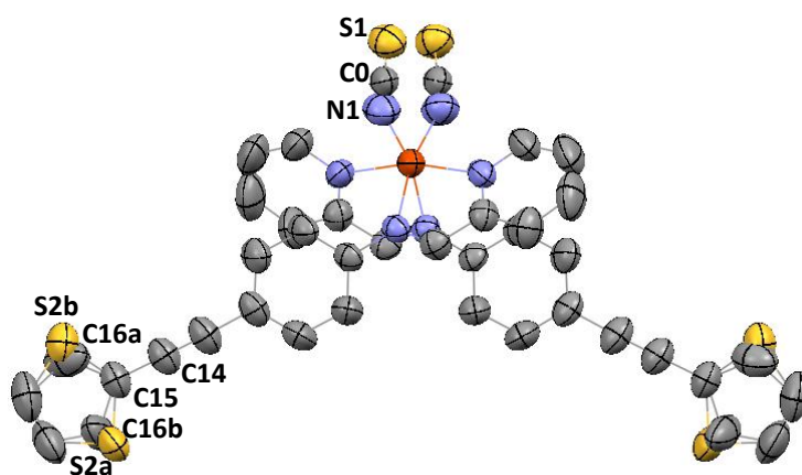
Figure 26 Fe-TheA-II : Structure moléculaire à 293K projetée selon l'axe b . Les ellipsoïdes sont à 50% de probabilité. Les atomes dont les paramètres d'agitation isotropes sont mentionnés dans le texte sont indiqués [Marchivie 2003].
